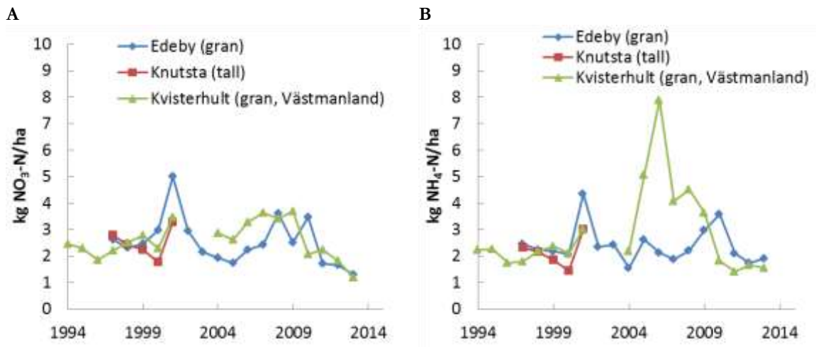
Figur 11. Årliga värden för nedfall av nitratkväve (A) och ammoniumkväve (B) med nederbörden till öppet fält till mätplatser i Södermanlands län samt Kvisterhult i södra Västmanland. Nedfallet är summerat som hydrologiskt år (okt-sept).
