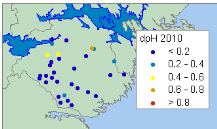
Figur 9. pH-förändring sedan förindustriell tid (dpH) i sjöar 2010, baserat på MAGIC-biblioteket. En sjö räknas som antropogent försurad om pH som årsmedian har sjunkit med minst 0,4 enheter sedan förindustriell tid (dpH > 0,4), vilket markeras med gula, orange och röda symbolerna på kartan. Analysen inkluderar kalkade försurade sjöar baserat på beräknad vattenkemi om man inte hade kalkat.
