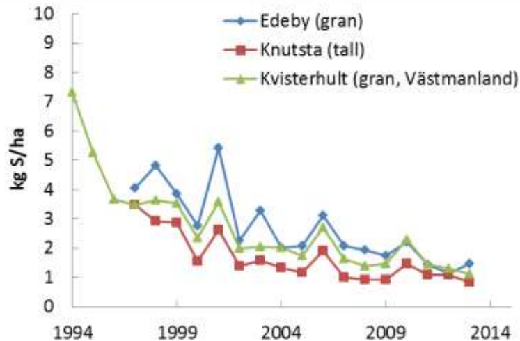
Figur 5. Svavelnedfall i granskogen vid Edeby i mellersta Södermanlands län, i tallskogen vid Knutsta, i norra Södermanlands län, samt i granskogen vid Kvisterhult i södra Västmanlands län. Svavelnedfallet med krondroppet har minskat signifikant vid samtliga tre mätplatser.
