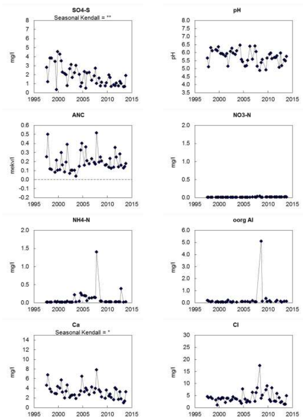
Figur B1:4. Markvattenkemi vid Knutsta, D 14 . Sulfatsvavel (SO 4 -S); pH; markvattnets syraneutraliserande förmåga (ANC); nitratkväve (NO 3 -N); ammoniumkväve (NH 4 -N); oorganiskt aluminium (oorg Al); kalciumhalt (Ca 2+ ) samt klorid (Cl). Saknade värden innebär oftast att marken varit för torr. Trendanalys har genomförts med hjälp av Seasonal- Kendall metodik och signifikansnivåer anges, ovanför respektive diagram, i de fall där signifikanta trender påvisats.
