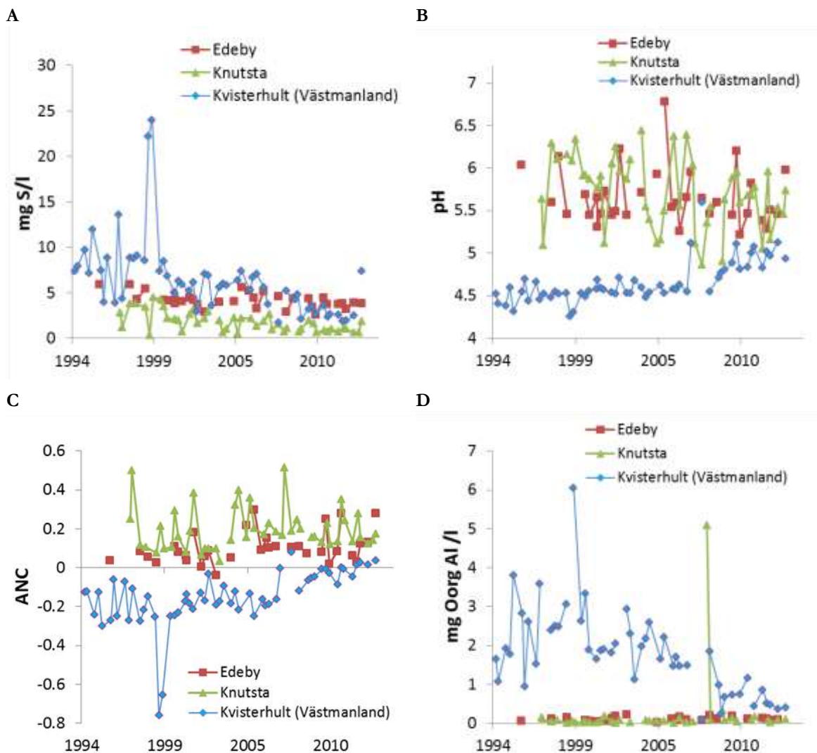
Figur 7. Halterna av sulfatsvavel (A, SO 4 -S), pH (B), syraneutraliserande förmåga (C, ANC) och halten oorganiskt aluminium (D, oorg-Al) i markvattnet på 50 cm djup vid olika platser i Södermanlands samt Västmanlands län, uppmätt inom Krondropps nätet. Följande förändringar är statistiskt säkerställda: SO 4 -S har minskat signifikant vid Edeby, Knutsta och Kvisterhult; pH har ökat signifikant vid Kvisterhult; ANC har ökat signifikant vid Edeby och Kvisterhult och oorg-Al har minskat signifikant vid Kvisterhult.
