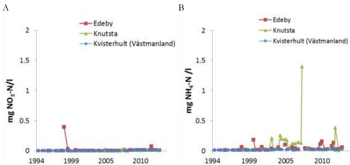
Figur 13. Halterna i markvattnet på 50 cm djup vid olika platser i Södermanlands län samt södra Västmanland av nitratkväve ( \text{NO}_3\text{-N} ) i markvattnet (A) samt halterna av ammoniumkväve ( \text{NH}_4\text{-N} ) i markvattnet (B). Inga förändringar är statistiskt säkerställda.
