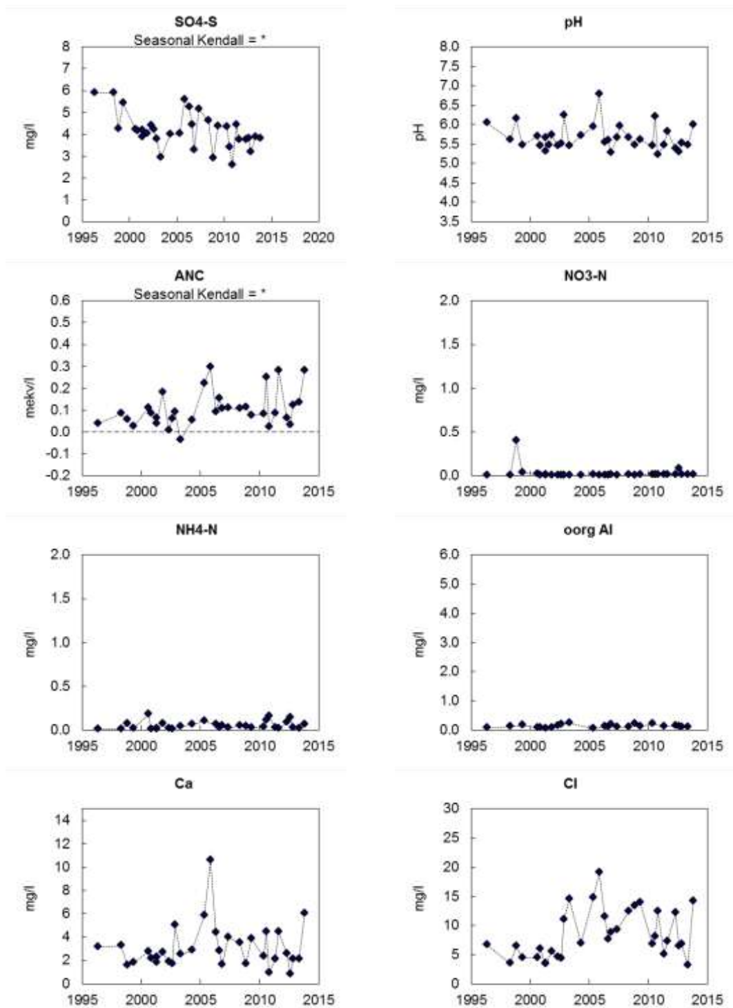
Figur B1.2. Markvattenkemi vid Edeby, D 11. Sulfatsvavel ( \text{SO}_4\text{-S} ); pH; markvattnets syraneutraliserande förmåga (ANC); nitratkväve ( \text{NO}_3\text{-N} ); ammoniumkväve ( \text{NH}_4\text{-N} ); oorganiskt aluminium (oorg Al); kalciumhalt ( \text{Ca}^{2+} ) samt kloridhalt (Cl). Saknade värden innebär oftast att marken varit för torr. Trendanalys har genomförts med hjälp av Seasonal-Kendall metodik och signifikansnivåer anges, ovanför respektive diagram, i de fall där signifikanta trender påvisats.
