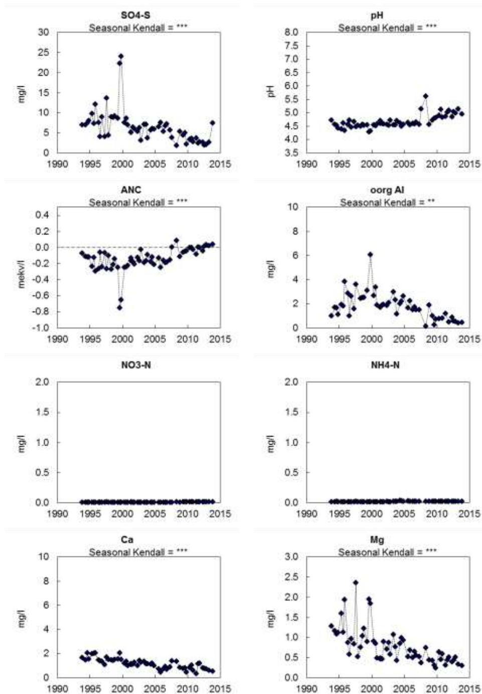
Figur B1:6. Markvattenkemi vid Kvisterhult, U 04: sulfatsvavel (SO 4 -S), pH, markvattnets syra-neutraliserande förmåga (ANC), oorganiskt aluminium (oorg Al), nitratkväve (NO 3 -N), ammoniumkväve (NH 4 -N), kalciumhalt (Ca 2+ ) och magnesiumhalt (Mg 2+ ). Sagnade värden innebär oftast att marken varit för torr. Observera att skalorna skiljer sig åt mot skalorna för Södermanlands egna mätlokaler. Trendanalys har genomförts med hjälp av Seasonal-Kendall och signifikans-nivåer anges, ovanför respektive diagram, i de fall där signifikanta trender påvisats.
