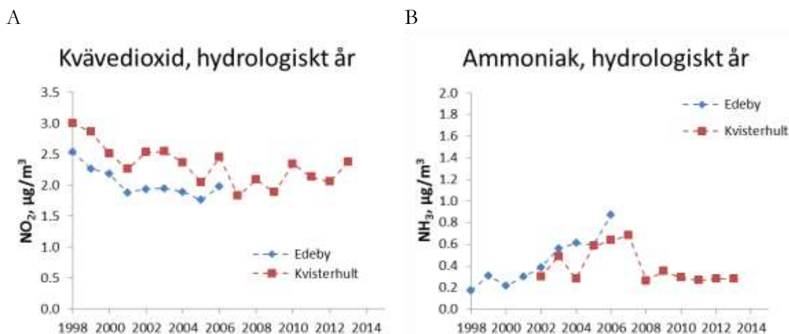
Figur 10. Lufthalter för kvävedioxid, \text{NO}_2 (A) och ammoniak, \text{NH}_3 (B) i Edeby (avslutades 2006) och i Kvisterhult i södra Västmanlands län. Lufthalterna av \text{NO}_2 minskar signifikant vid Kvisterhult enligt Mann-Kendall analys.
