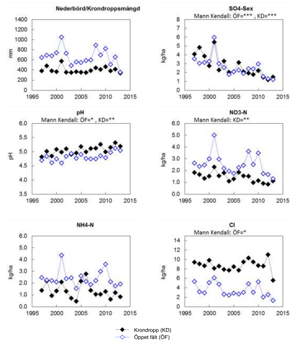
Figur B1:1. Årliga värden (hydrologiskt år) för depositionen via krondropp och över öppet fält vid Edeby, D 11 . I figuren visas uppmätt nederbörd över öppet fält samt krondroppsmängder, uttryckt som mm. Deposition redovisas sedan mätningarna påbörjades för ett urval av ämnen: sulfatsvavel utan havssaltsbidrag ( \text{SO}_4\text{-S ex} ), pH; nitratkväve ( \text{NO}_3\text{-N} ); ammoniumkväve ( \text{NH}_4\text{-N} ) samt kloridjoner ( \text{Cl} ). ÖF, öppet fält; KD, krondropp. Trendanalys har genomförts med hjälp av Mann-Kendall metodik och signifikansnivåer anges, ovanför respektive diagram, i de fall där signifikanta trender påvisats.
