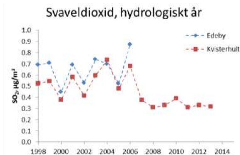
Figur 4. Svavelhalter i luften i Edeby (1998-2006) och i Kvisterhult i södra Västmanlands län. Lufthalterna av SO 2 minskar signifikant vid Kvisterhult enligt Mann-Kendall analys.
