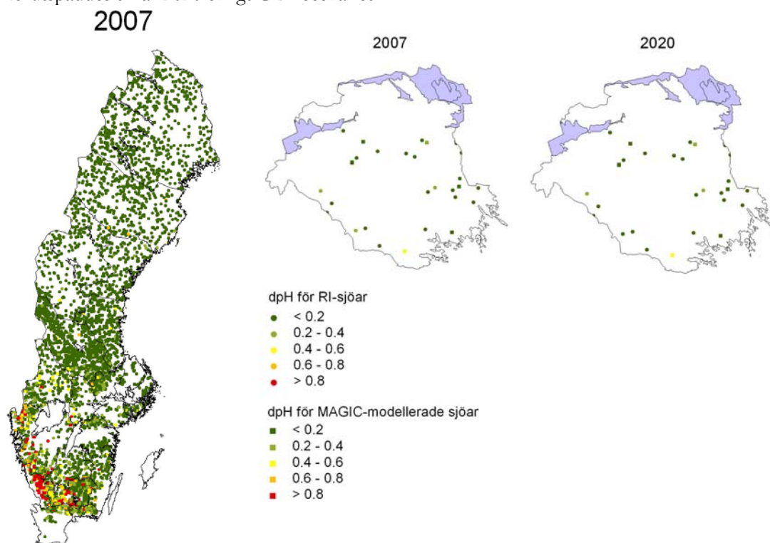
Figur 15. pH-förändring sedan förindustriell tid (dpH) i sjöar 2007 och 2020 (enligt CLE-scenariot), baserat på MAGIC. Fyrkanterna är sjöar modellerade med MAGIC-modellen, medan cirklarna är sjöar inom Riksinventeringarna som är bedömda enligt MAGIC-biblioteket, d.v.s. sjöar som inte är modellerade, utan jämförda med liknande modellerade sjöar. I de fall där en sjö är bedömd både baserat på Riksinventeringen 2000 och Riksinventeringen 2005 är det den senare som använts i kartan.
