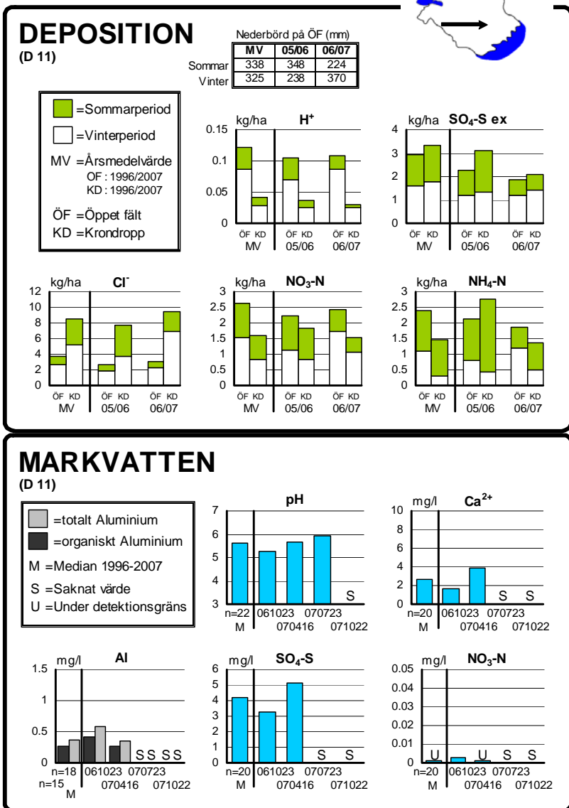
Figur 3. Depositions- och markvattendata från Edeby D 11. I figuren redovisas deposition av ett urval ämnen i öppet fält och i kronddropp de två senaste åren och jämförs med ett medelvärde för perioden 1996-2007 för öppet fält och kronddropp. Åren är indelade i sommar- (april-sep) och vinterperiod (okt-mars). För markvatten redovisas det senaste årets provtagningar, vilka jämförs med ett långtidsvärde. Medianvärde används för att undvika en kraftig inverkan av enstaka höga halter som ibland uppträder under torra förhållanden. Saknade värden innebär oftast att marken varit för torr. Al är uppdelat i total och organisk halt. Skillnaden utgör oorganiskt Al som i höga halter medför risk för skador på känsliga organismer i mark och vatten. Kemiska beteckningar som används i figurerna är vätejoner ( H^+ ), sulfatsvavel utan havssaltsbidrag ( SO_4\text{-S}_{ex} ), sulfatsvavel ( SO_4\text{-S} ), kloridjoner ( Cl^- ), nitratkväve ( NO_3\text{-N} ), ammoniumkväve ( NH_4\text{-N} ), kalciumjoner ( Ca^{2+} ) och aluminium ( Al ).
