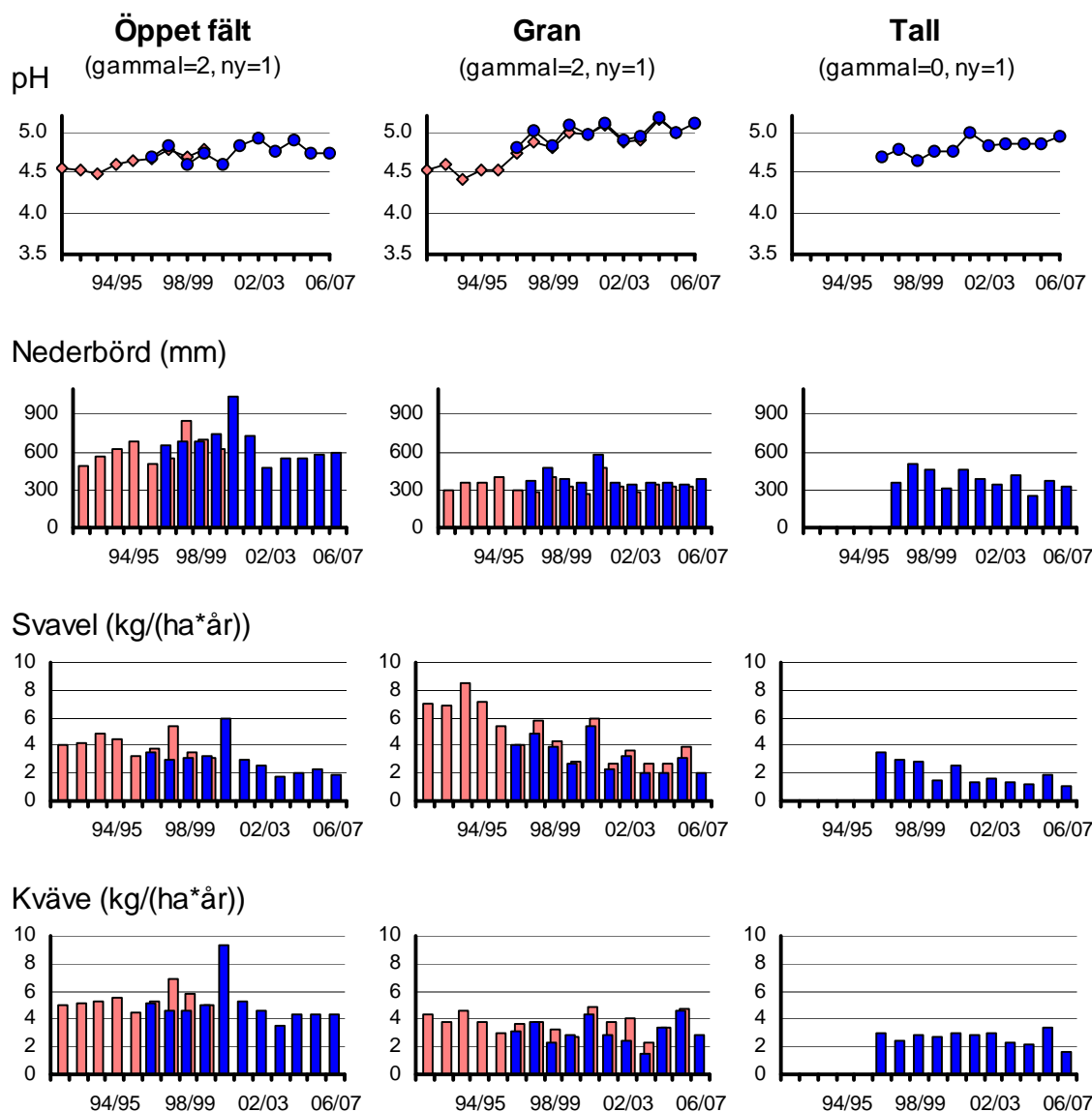
Figur 6. Årsmedelvärden för pH, nederbörd, deposition av svavel och oorganiskt kväve i tre miljöer i Södermanlands län; öppet fält, granskog och tallskog, uppdelat på två tidsserier. För "gammal" tidsserie för både öppet fält och granytan har mätningar från Åker och Råsjön (1991-2000) använts och för "ny" tidsserie för både öppet fält och granytan har mätningar från Edeby (1996-2007) använts. För tallytan finns endast en "ny" tidsserie och den omfattar mätningar från Knutsta mellan 1996-2007.
