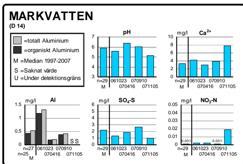
Figur 5. Markvattendata från Knutsta, D 14. I figuren redovisas resultaten från det senaste årets tre provtagningar, vilka jämförs med ett långtidsvärde. Medianvärde används för att undvika en kraftig inverkan av enstaka höga halter som ibland uppträder under torra förhållanden. Saknade värden innebär oftast att marken varit för torr. Al är uppdelat i total och organisk halt. Skillnaden utgör oorganiskt Al som i höga halter medför risk för skador på känsliga organismer i mark och vatten. Kemiska beteckningar som används i figurerna är kalciumjoner (Ca 2+ ), aluminium (Al + ), sulfatsvavel (SO 4 -S) och nitratkväve (NO 3 -N).
