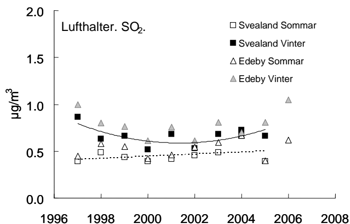
Figur 8. Lufthalter av SO 2 i Södermanlands län och för Svealand, redovisat som periodmedelvärden uppdelade på sommar- och vinterhalvår. Värdena baseras på månadsvisa mätningar och utgör medelvärden för en mätplats i Södermanlands län, Edeby, och fyra mätplatser för Svealand som helhet, varav Edeby utgör en mätplats. Trendlinjer visas för perioden 1998-2005 för Svealand sommarhalvår (streckad linje) och Svealand vinterhalvår (heldragen linje). Trendanalyserna som baseras sig på en polynomfunktion har en korrelationskoefficient för Svealand vintervärden på 0,47 och för Svealand sommarvärden på 0,13. Motsvarande värden för en linjär funktion blir 0,04 och 0,13 för vinter och sommar värden. Beräkningarna gäller kalenderår, sommar (april-september), vinter (jan-mars, okt-dec).
