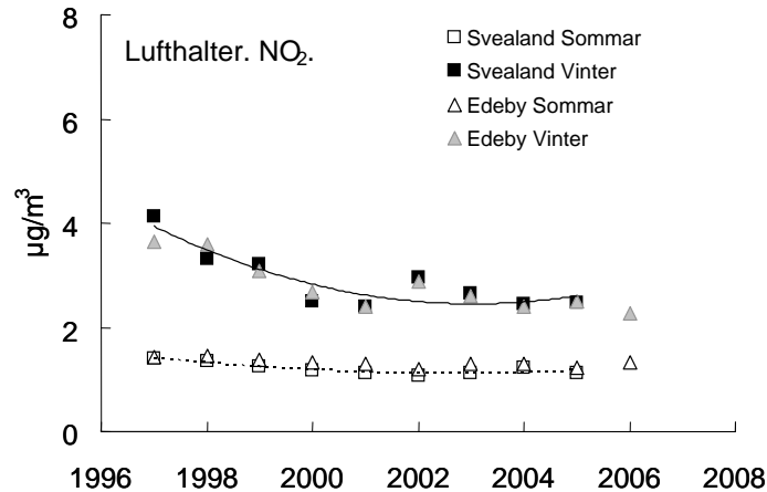
Figur 9. Lufthalter av NO 2 för Södermanlands län och för Svealand, redovisat som periodmedelvärden uppdelade på sommar- och vinterhalvår. Värdena baseras på månadsvisa mätningar och utgör medelvärden för en mätplats för Södermanlands län, Edeby, och fyra mätplatser för Svealand som helhet, varav Edeby utgör en mätplats. Trendlinjer visas för perioden 1997-2005 för Svealand sommarhalvår (streckad svart linje) och Svealand vinterhalvår (heldragen svart linje). Trendanalyserna som baserar sig på en polynomfunktion har en korrelationskoefficient för Svealand vintervärden på 0,81 och för Svealand sommarvärden på 0,82. Motsvarande värden för en linjär funktion blir 0,62 och 0,55 för vinter och sommar värden. En polynomfunktion beskriver således trenderna i data bättre än en linjär funktion. Beräkningarna gäller kalenderår, sommar (april-september), vinter (jan-mars, okt-dec).
