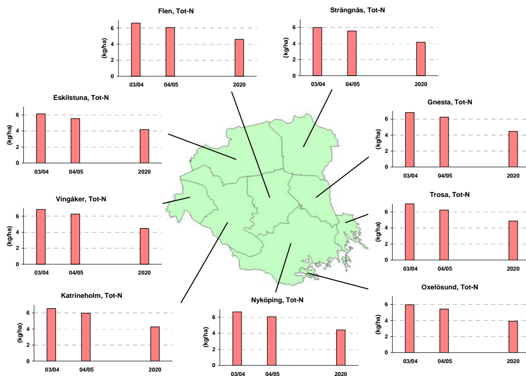
Figur 13. Kvävenedfall på kommunnivå i Södermanlands län under de hydrologiska åren 2003/04, 2004/05 och år 2020 enligt CLE-scenariet, modellerat med MATCH-Sverige modellen.
