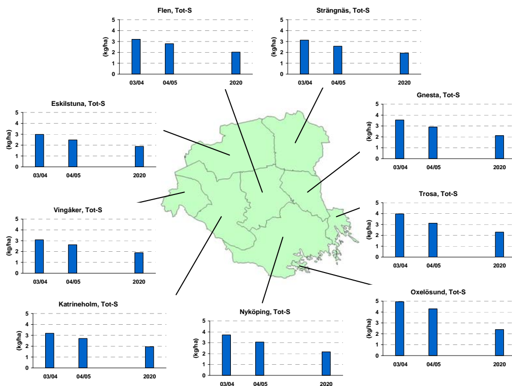
Figur 12. Svavelnedfall på kommunnivå i Södermanlands län under de hydrologiska åren 2003/04, 2004/05 och år 2020 enligt CLE-scenariet, modellerat med MATCH-Sverige modellen.
