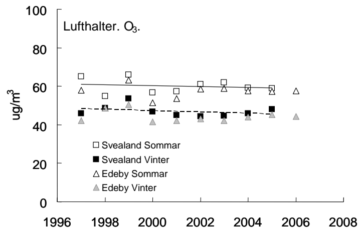
Figur 11. Lufthalter av ozon som medelvärde för Södermanlands län och som medelvärde för Svealand, redovisat som periodmedelvärden uppdelat på sommar- och vinterhalvår. Värdena baseras på månadsvisa mätningar och utgör medelvärden för en mätplats i Södermanland, Edeby, och fyra mätplatser för Svealand som helhet, varav Edeby utgör en mätplats. Trendlinjer visas för perioden 1997-2005 för Svealand sommarhalvår (heldragen linje, minskning 0,2 µg/m 3 årligen) och Svealand vinterhalvår (streckad linje, minskning 0,3 µg/m 3 årligen). Beräkningarna gäller kalenderår, sommar (april-september), vinter (jan-mars, okt-dec).
