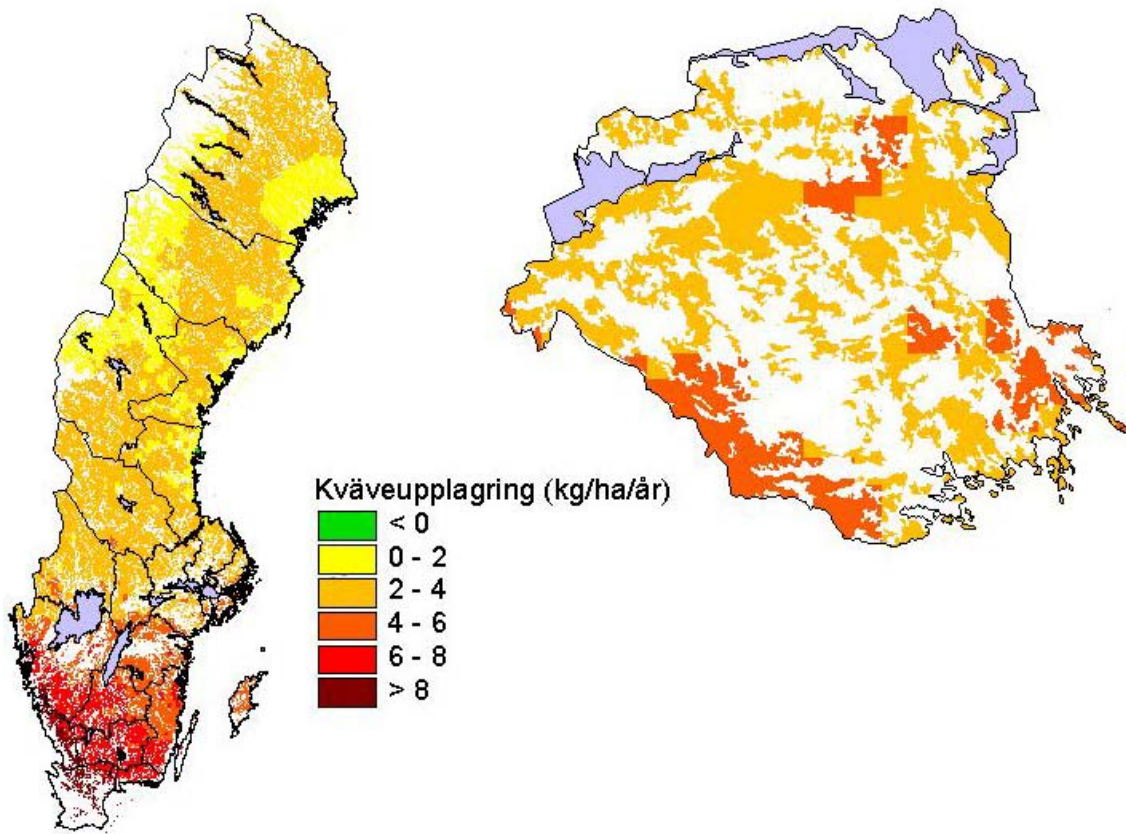
Figur 16. Kväveackumulering i granskog i Sverige och i Södermanland. Färgade områden är alla typer av skogsmark medan vita områden är mark med annan markanvändning. Kväveupplagringen som anges gäller enbart granskog.
