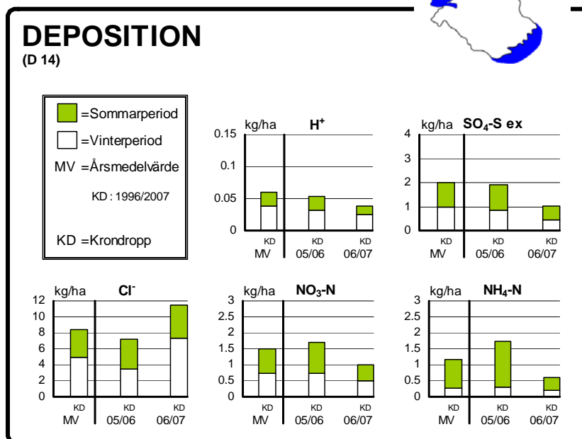
Figur 4. Depositionsdata från Knutsta, D 14. I figuren redovisas deposition av ett urval ämnen i krondropp de två senaste åren och jämförs med ett medelvärde för perioden 1996-2007 för både öppet och krondropp. Åren är indelade i sommar- (april-sep) och vinterperiod (okt-mars). Kemiska beteckningar som används i figurerna är vätejoner (H + ), sulfatsvavel utan havssaltsbidrag (SO 4 -Sex), kloridjoner (Cl - ), nitratkväve (NO 3 -N) och ammoniumkväve (NH 4 -N).
