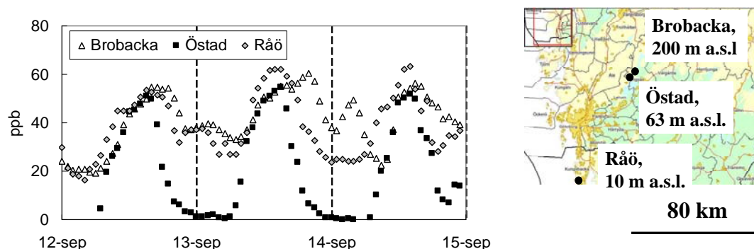
Figur 18. En sekvens med mätningar av ozonhalter med instrument vid tre olika platser i Västsverige som timmedelvärden under tre dagar med högtrycksbetonat väder i september 2006. Råö är en permanent mätplats inom EMEPs nätverk, belägen ca 40 km söder om Göteborg precis vid kusten. Östads Säteri är en mätplats som drivs av IVL Svenska Miljöinstitutet och Göteborgs Universitet, belägen topografiskt lågt i landskapet, ca 50 km nordost om Göteborg. Brobacka är en tillfällig mätplats, belägen på toppen av ett berg, högt över omgivande landskap, ca 8 km nordost om Östads Säteri. a.s.l. betecknar höjd över havet.
