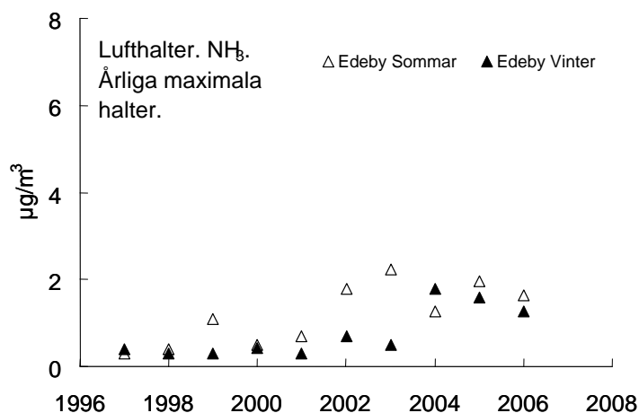
Figur 10. Lufthalter av ammoniak för Södermanlands län, som årliga maximala värden uppdelat på sommar och vinterhalvår. Värdena baseras på månadsvisa mätningar vid en mätplats i länet, Edeby. Beräkningarna gäller kalenderår, sommar (april-september), vinter (jan-mars, okt-dec).
